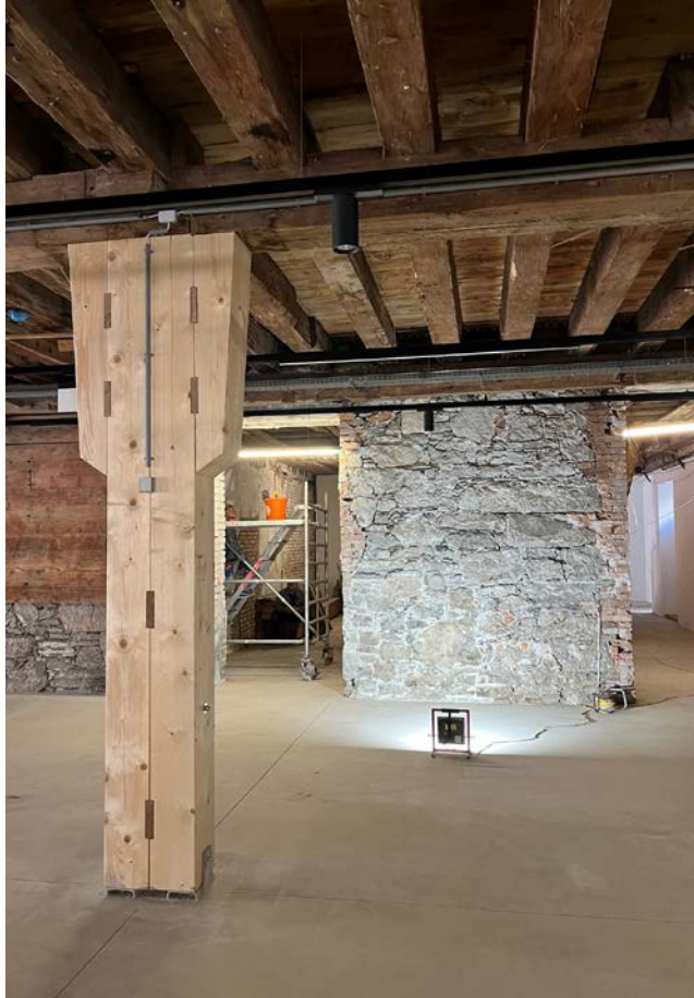
Alte Saline Hallein, Adaptierung zum Kultur- und Veranstaltungsort
